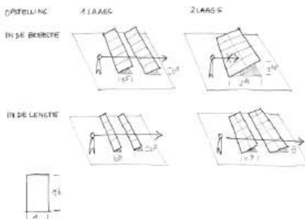
Opstellingsmogelijkheden panelen van 1 x 1,5 meter en de relatie met zicht en beschadwing van de bodem
