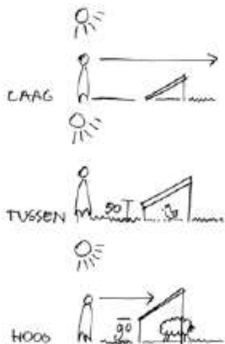
Relatie tussen constructiehoogte, zicht en dubbel grondgebruik
